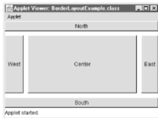
BorderLayout
