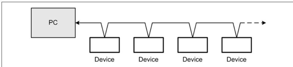
Figure 7-26. RS-485 multidrop
