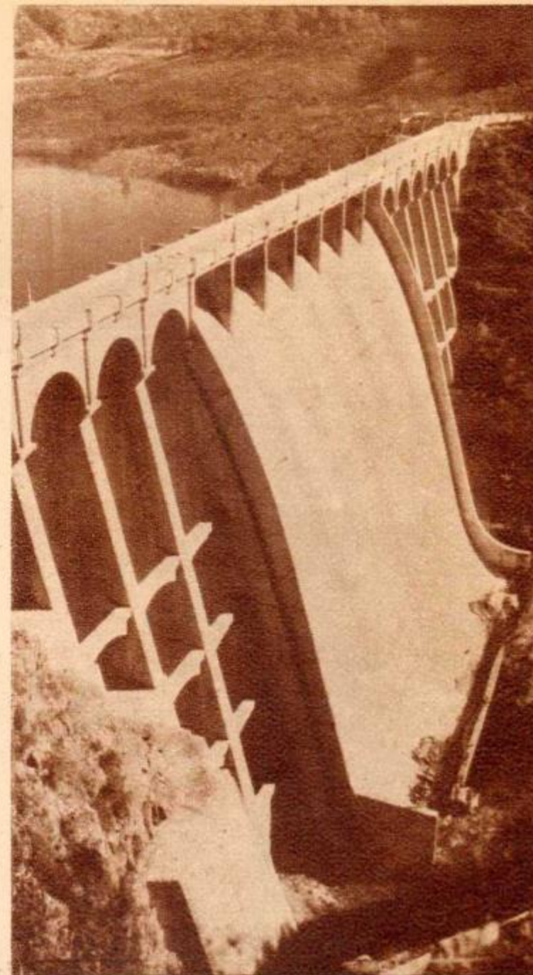
El dique Escaba, construido en la provincia de Tucumán, sobre el río Marapa, costó cincuenta millones de pesos y permite la irrigación de 29.500 hectáreas de tierra.
